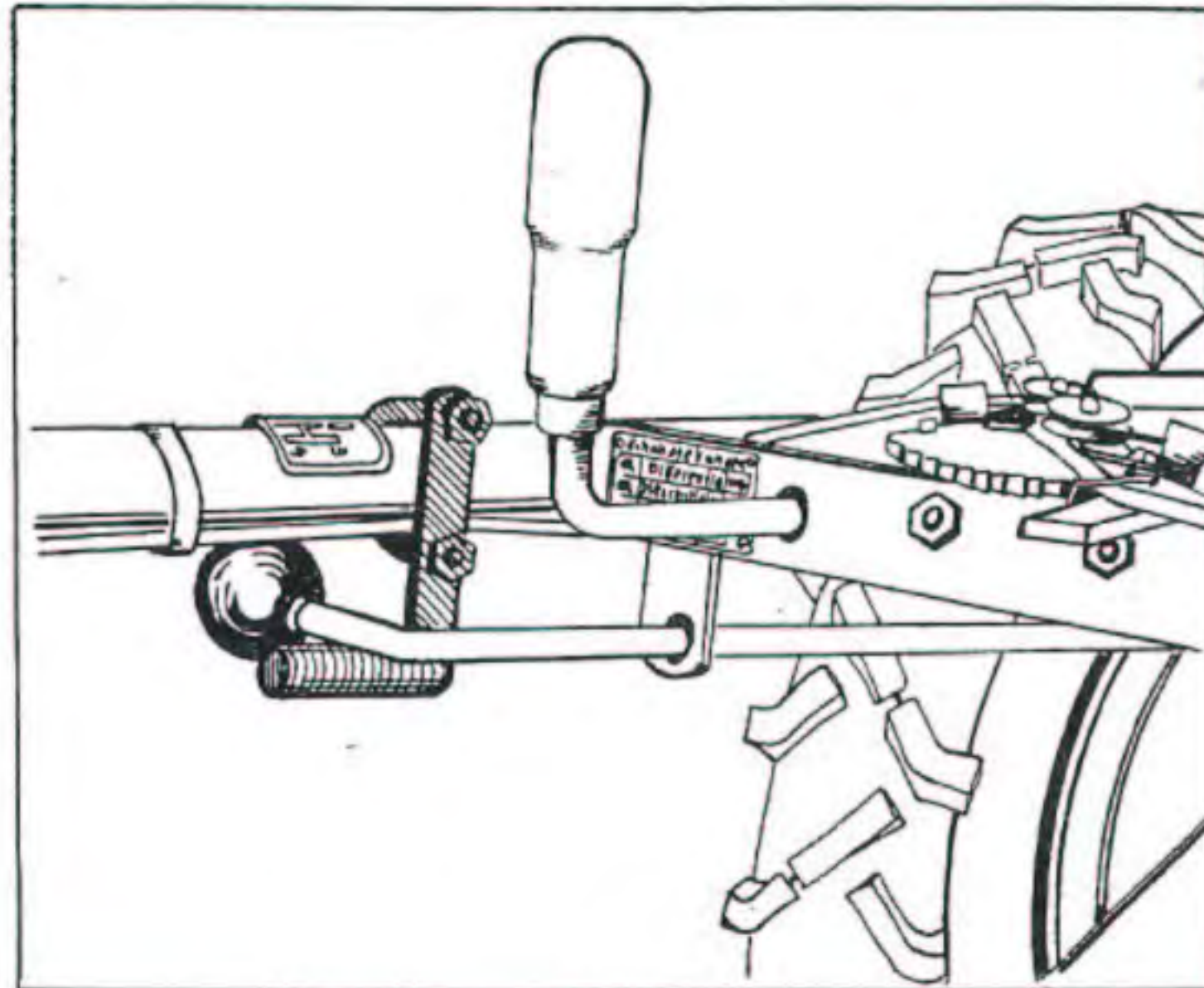
Sperre für Drehgrifflenkung beim Einachsräumer BED II
