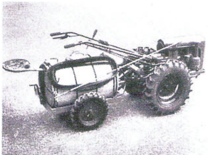
mit HOLDER-Zweikolben-Pumpe und Faßwagen 200 Liter Inhalt
