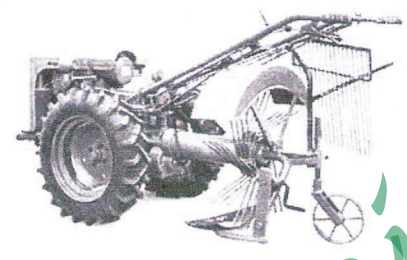
mit Zapfwellen-Kartoffelschleuderräder
