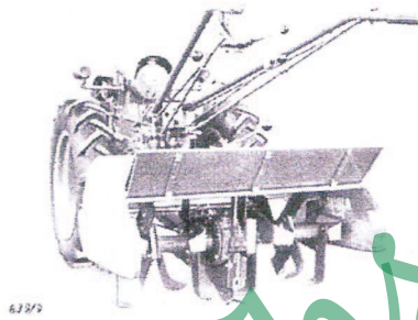
mit Anbau-Hackfräse (Rotorhacke) (Arbeitsbreiten 70–185 cm)
