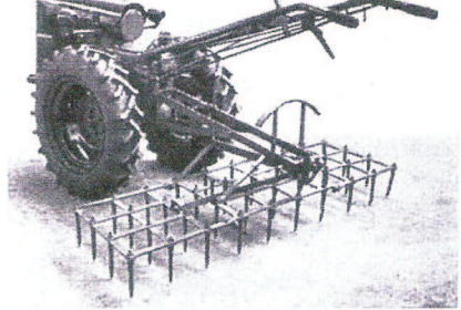
mit Anbauegge (Arbeitsbreite 1,8 m)
