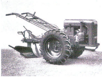
mit Geräterahmen und Drehpflug
