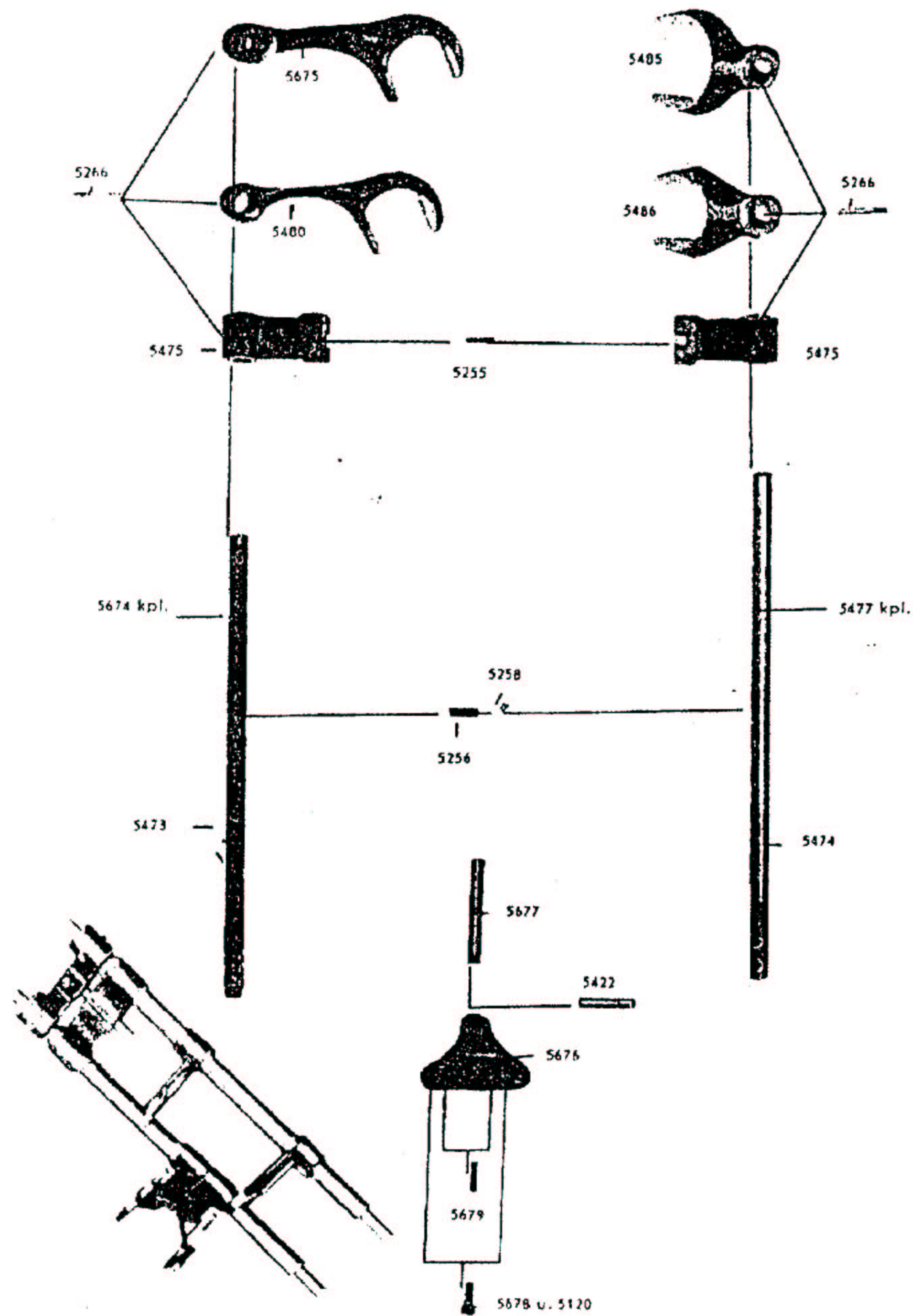
5673 Schaltwerk kpl.
